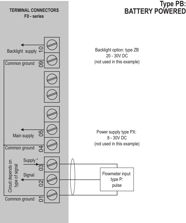
Configuration example F011-P-PB-(PX)-(XX)-(ZB)
